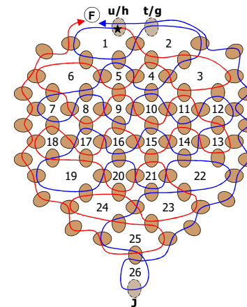
Skizze 5: Flügel (2x)
